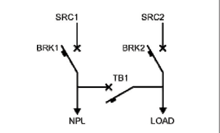
CASO C: 2S - 1T - SI
