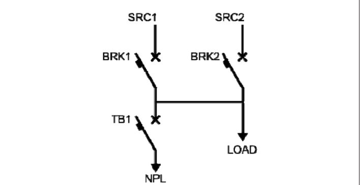
CASO O: 2S-NPL
