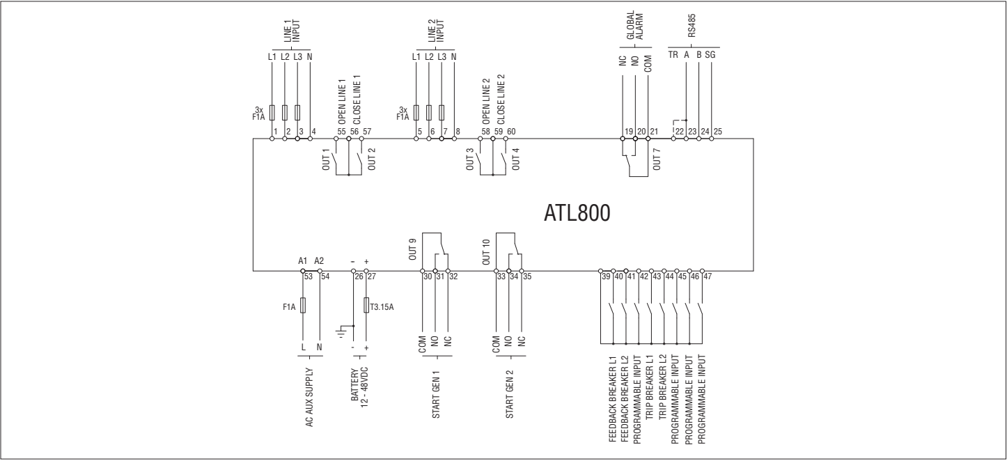
SCHEMA POTENZA CON INTERRUTTORI
