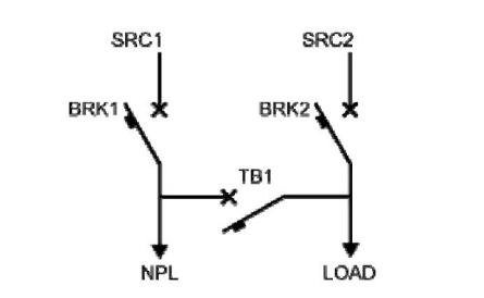
CASO B: 2S - 1T - PL
