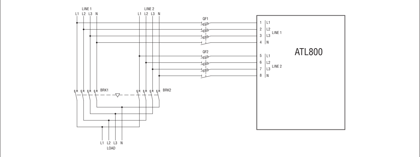
SCHEMA POTENZA CON INTERRUTTORI
