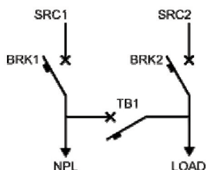
CASE B: 2S – 1T – PL
