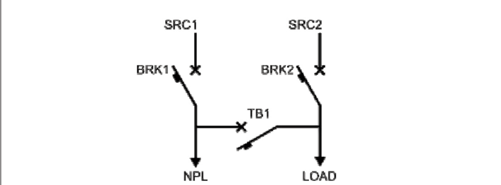
CASO D: 2S - LT - AL
