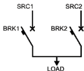
CASE A: 2S – 0T
