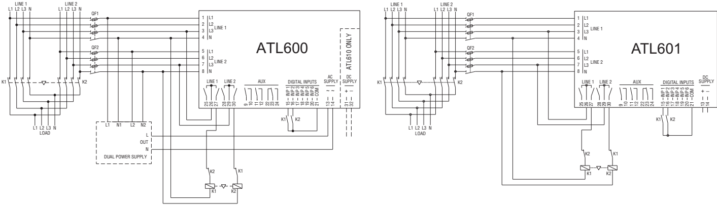
Parameter setting for the wiring diagram in picture Programmazione parametri per lo schema in figura
