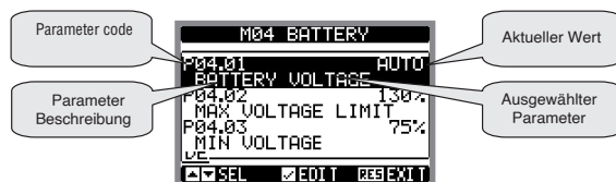
Einstellung: Parameterauswahl
