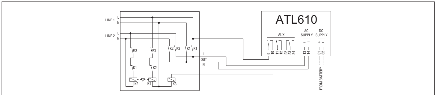
Empfohlene Ausführung für Anwendungen mit Notstromaggregaten Netz 2 vom Generator kommend Kontrolle der Hilfsspannung mittels ATL610 + AC Dual Power Supply (optional) (Anlage mit Stromversorgung von Akku)
