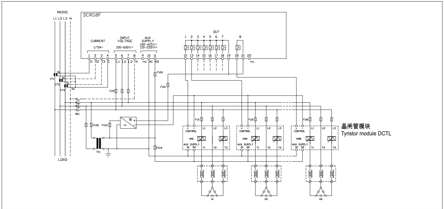
晶闸管模块使用干结点进行控制 (仅适用于晶闸管模块 DCTL 系列)
