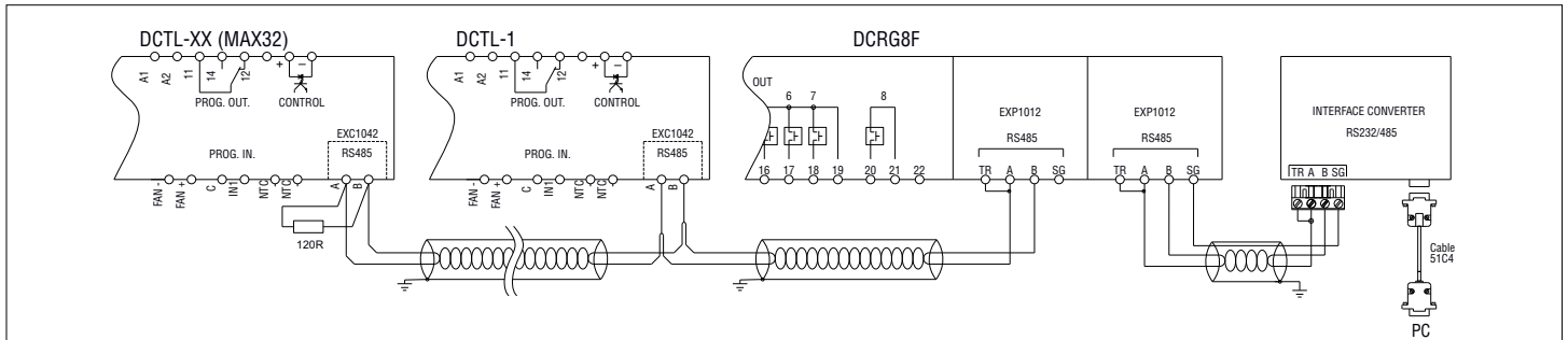
经由 RS485 总线控制晶闸管模块 (仅适用于晶闸管模块 DCTL 系列)
