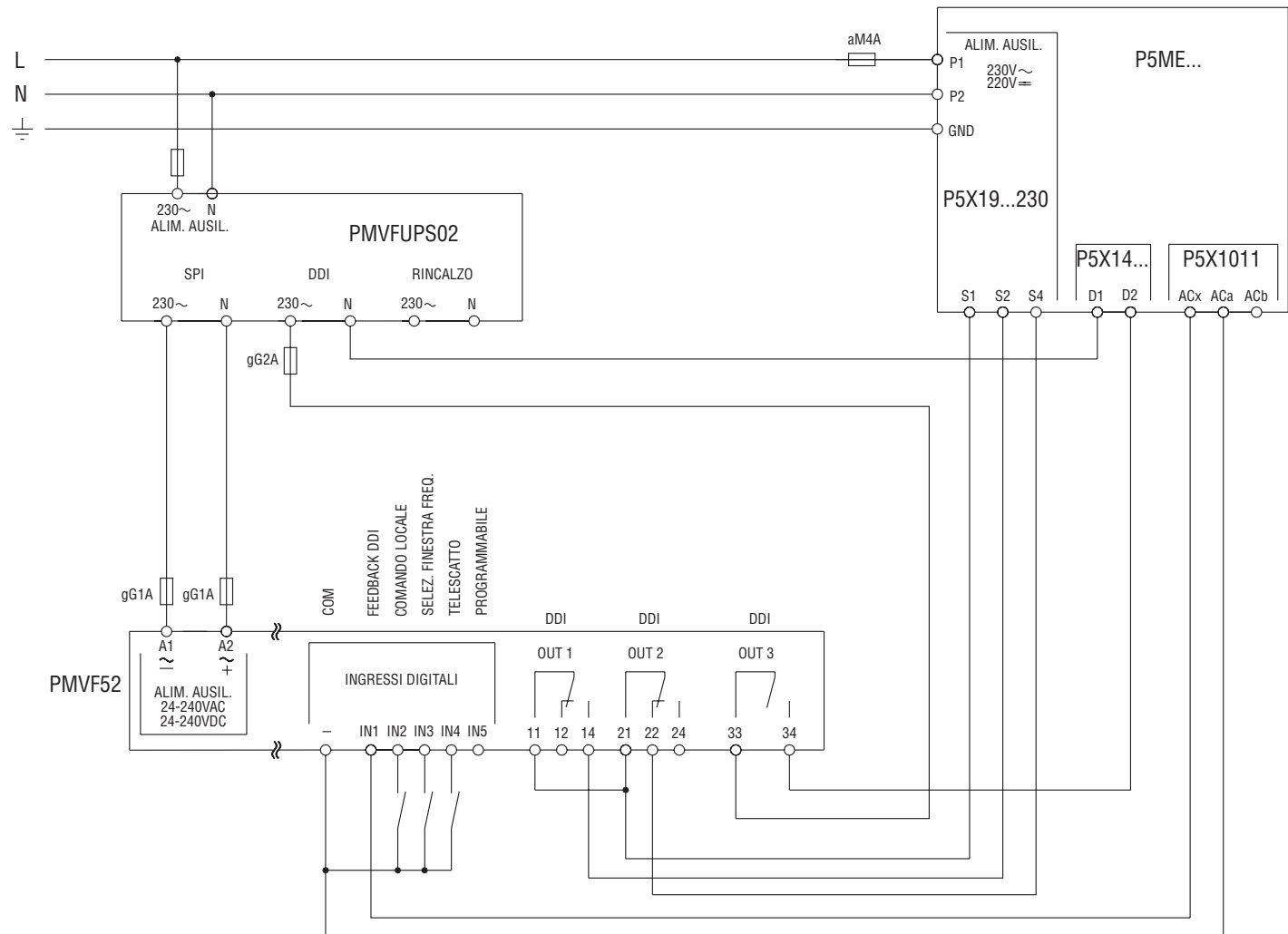
ESEMPIO 4: Configurazione con due uscite separate per il controllo dell'apertura e della chiusura e un'ulteriore uscita (OUT3) per la gestione della bobina di minima tensione.
