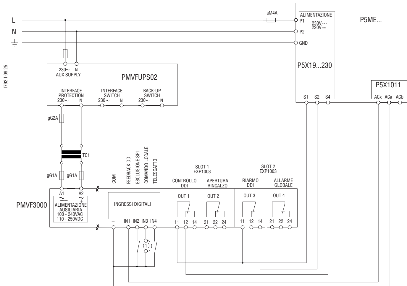
ESEMPIO 6: Configurazione con due uscite distinte comandanti l'apertura e la chiusura per interruttori scatolati con comando impulsivo.
