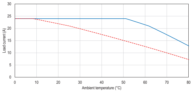
HS3D5HV024E230
