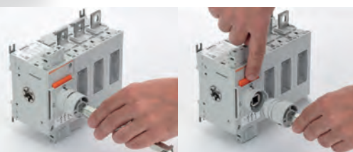
Montaż i demontaż zatraskowego trzpienia
