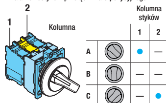
Działanie zestawów przełącznika 3 pozycyjnego
