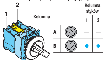
Działanie zestawów przełącznika 3 pozycyjnego
