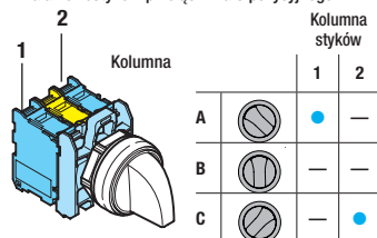
Działanie zestyków przełącznika 3 pozycyjnego
