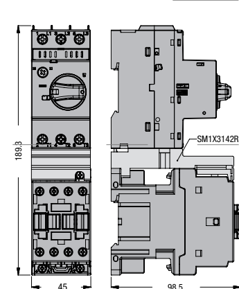
SM1R... ze stycznikiem BF09D...BF25D... lub BF09L...BF25L... i złączem SM1X3142R
