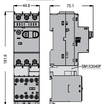
SM1P... ze stycznikiem BG... i złączem SM1X3040P
