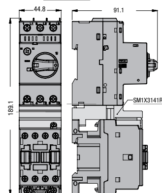
SM1R... ze stycznikiem BF09A...BF25A... i złączem SM1X3141R
