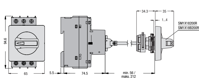
SM1R... z pokrętkiem SM1X18200R lub SM1X18B200R
