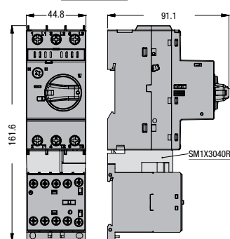
SM1R... ze stycznikiem BG... i złączem SM1X3040R
