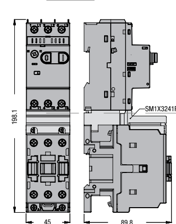
SM1P... ze stycznikiem BF26A...BF38A... i złączem SM1X3241P
