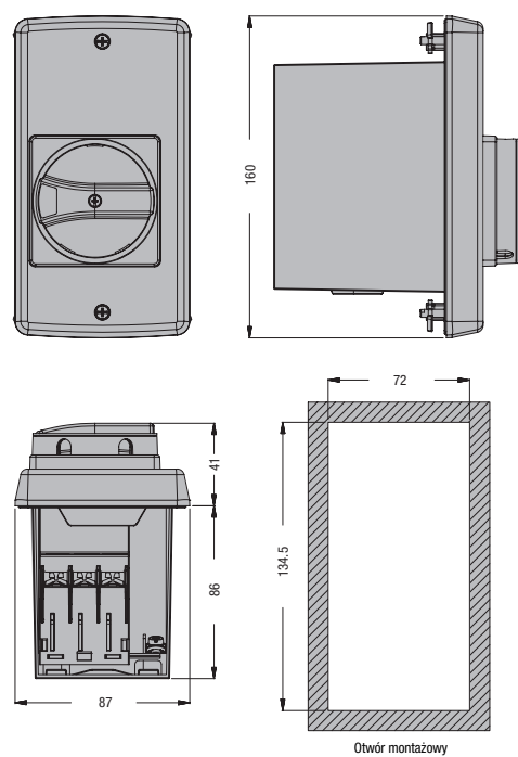
Obudowy SM1Z1720R i SM1Z1725R
