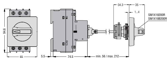
SM1R... con maniglia blocco porta lucchettabile SM1X18200R o SM1X18B200R
