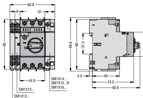
SM1R... con contatti ausiliari laterali
