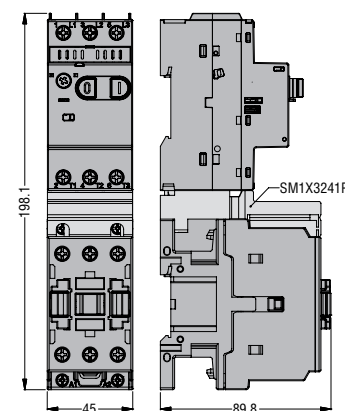
SM1P... con contattori BF26A...BF38A... e connessione SM1X3241P
