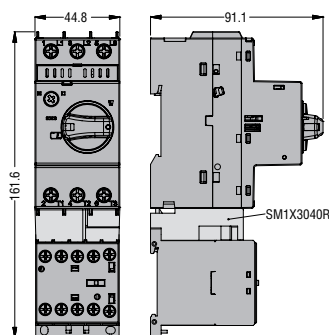
SM1R... con minicontattori BG... e connessione SM1X3040R
